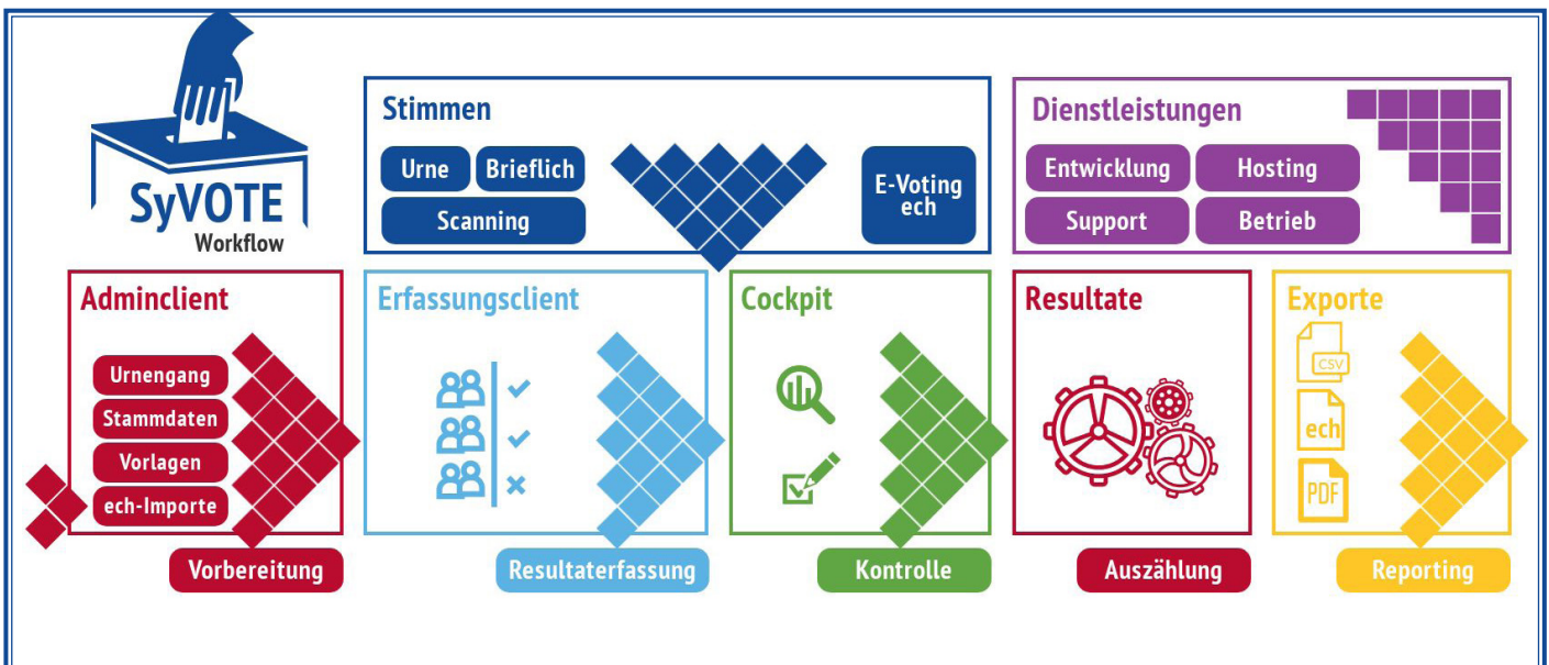
SyVOTE Prozess
